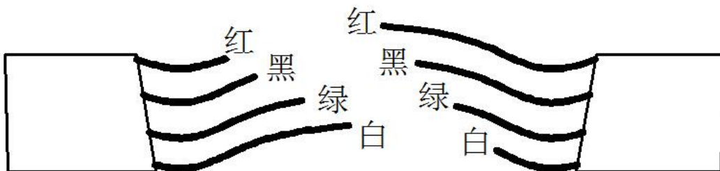
图 5-1 轴力计接线示意图
