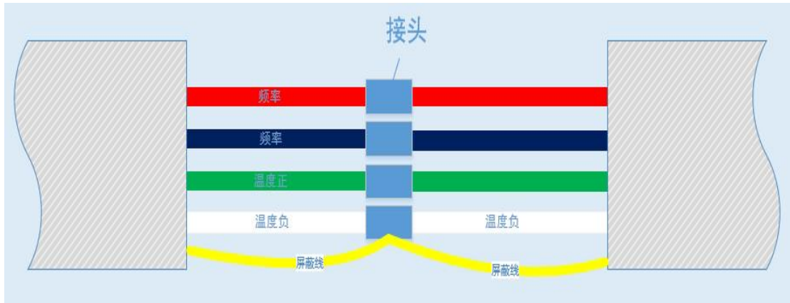
图 5-2 轴力计连接方式示意图
