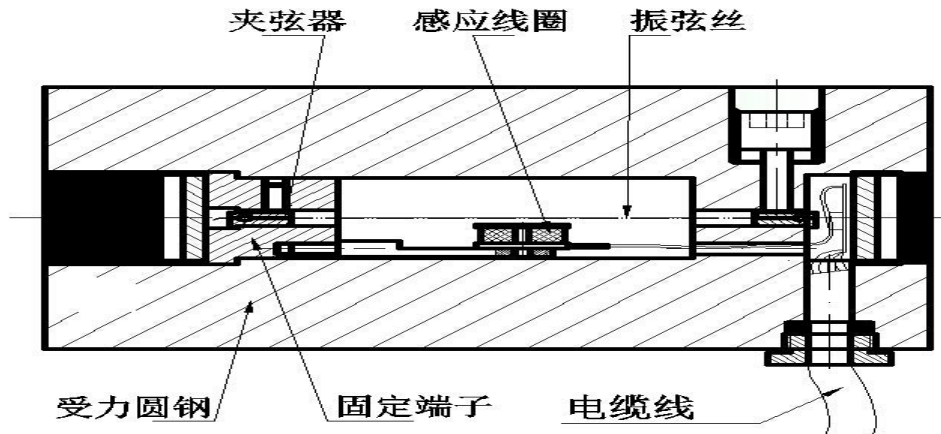
图 2-1 轴力计内部结构图
